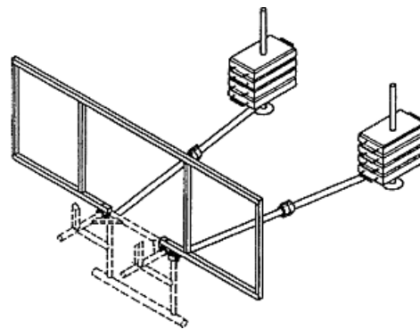
Flachdachbefestigung mit Ballastgewichten, Grundrahmen und Schutzgerüst Skizze 3.2
