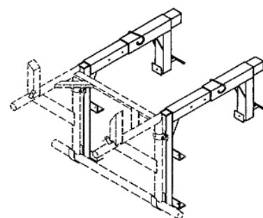
Fensterbefestigung mit Grundrahmen Skizze 1.2
