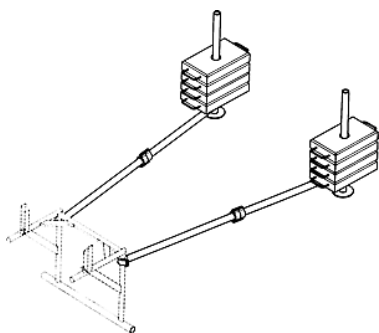
Flachdachbefestigung mit Ballastgewichten und Grundrahmen Skizze 3.1
