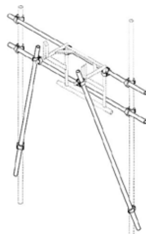
Beispiel für die Schuttrutschen Aufhängung am Gerüst (Feldlänge 2,5 m) Skizze 1.1
