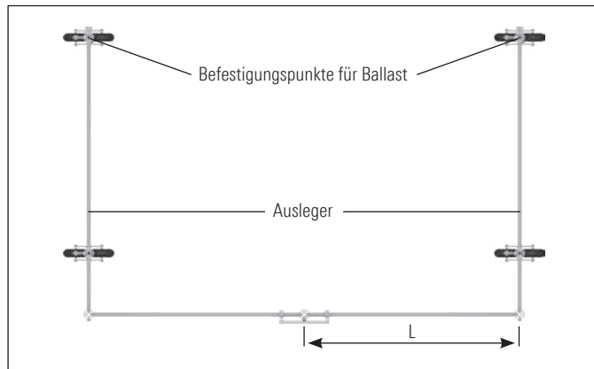
Draufsicht
