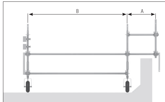
Seitenansicht
